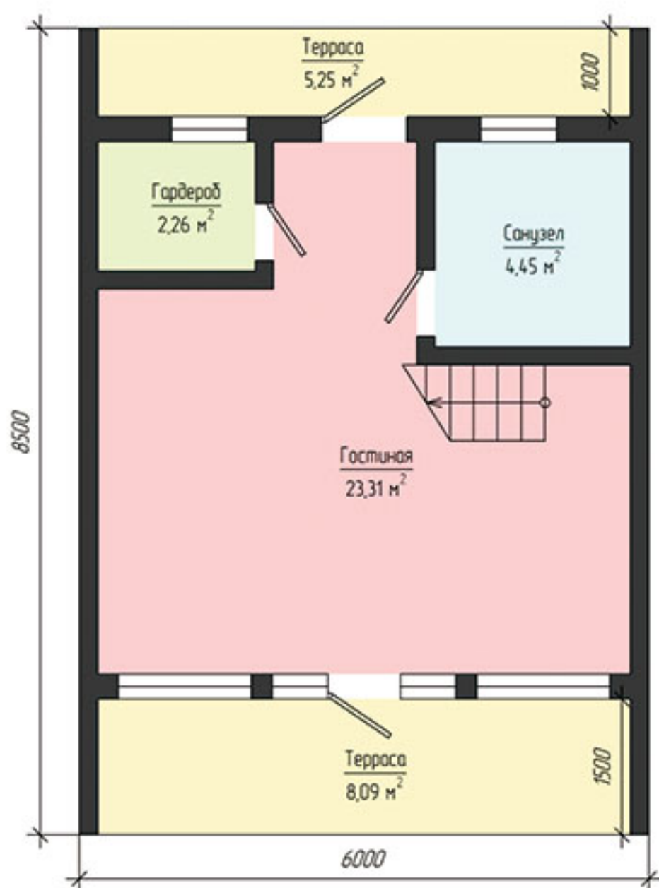
Этаж 1
