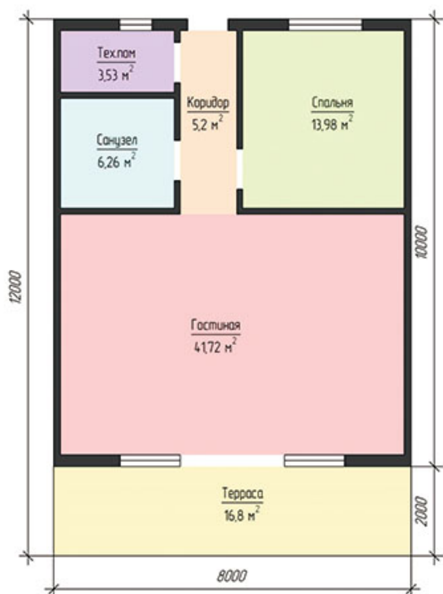
Этаж 1
